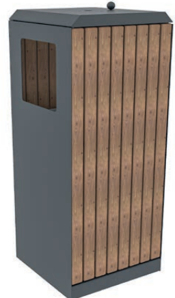
Ürün Ölçüleri : 35x35x90 Dimensions (cm)
