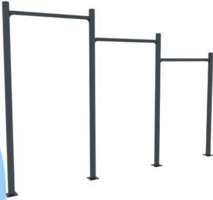
Ürün Ölçüleri : 400x35x250 Dimentions (cm)
