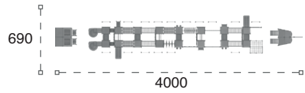
28 A Gemi Temalı Ahşap Oyun Grubu Ship Themed Wooden Playground
